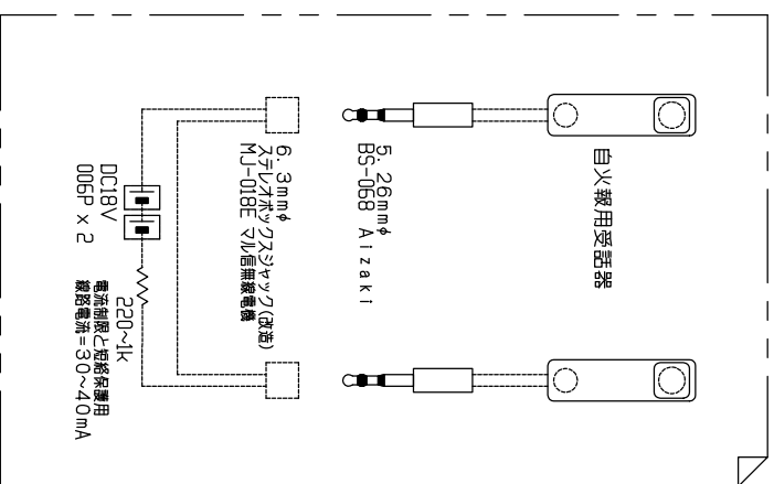
自火報用受話器之台での接続例
